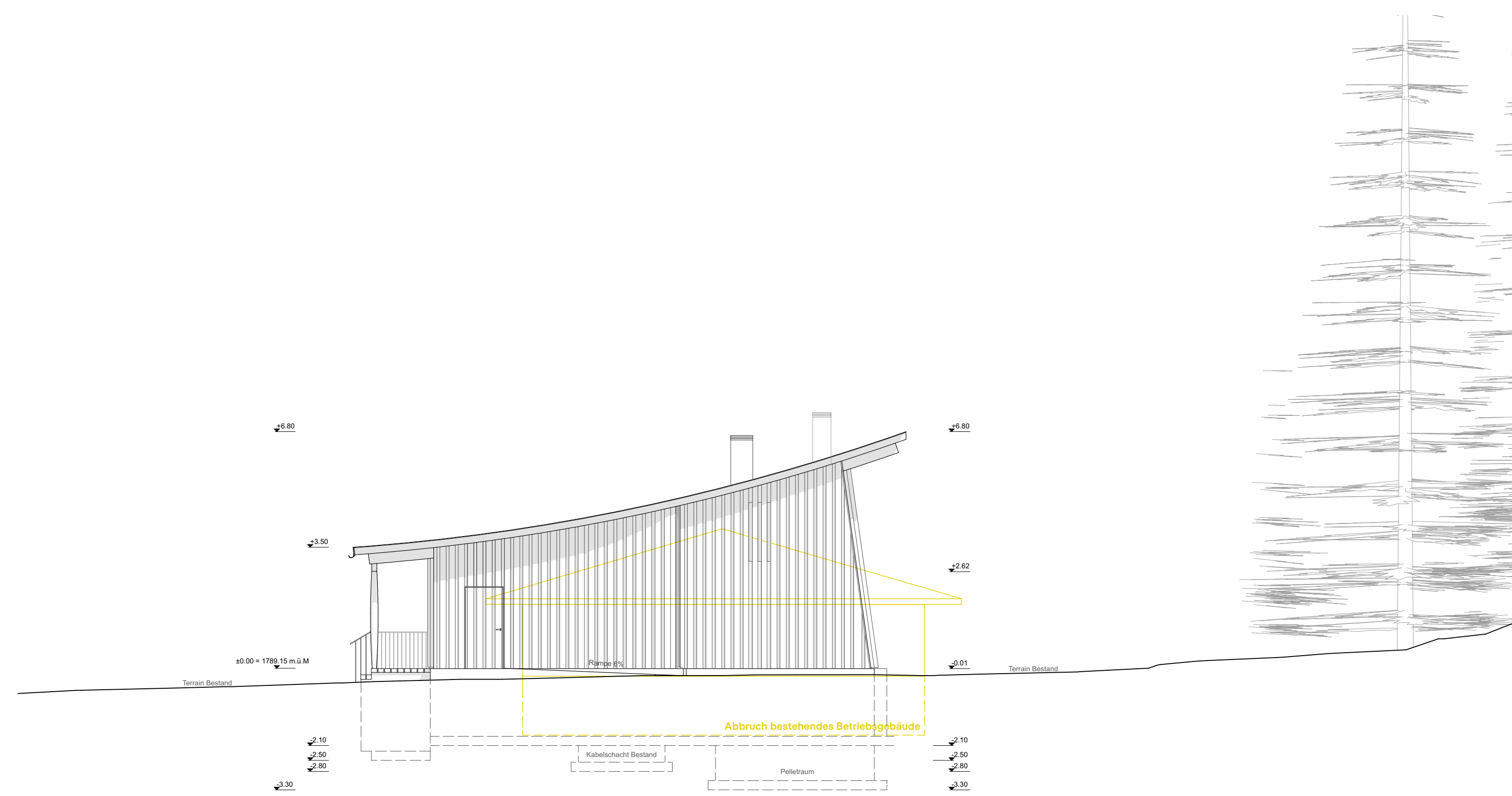
Ansicht Nord
